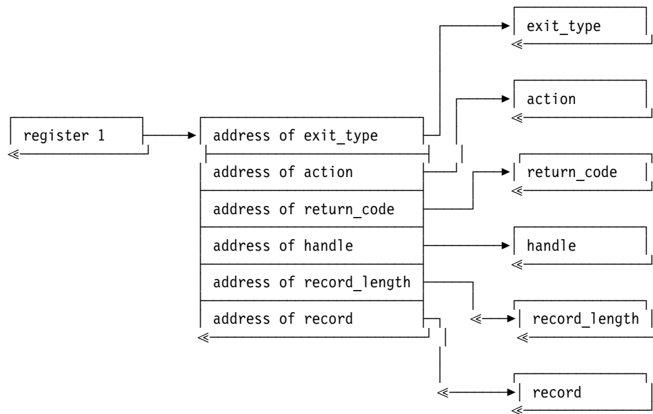
Figure 85. Filter module parameter list format
