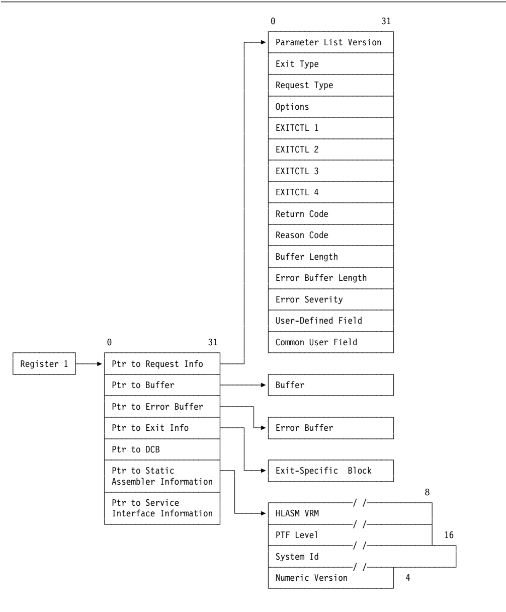
Figure 22. Exit parameter list format
